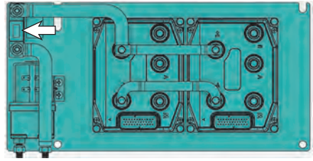
메인 퓨즈 - 48V 500 A
